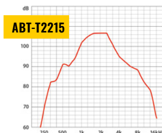
Frequenzgang:
