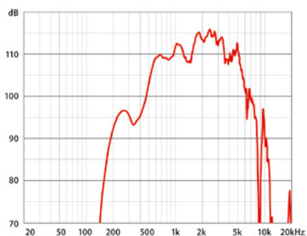
Frequenzgang:
