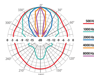
Polardiagramm Richtcharakteristik:
