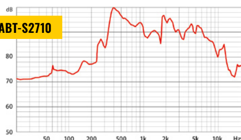
Frequenzgang:
