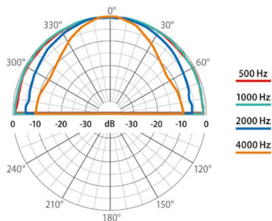
Polardiagramm Richtcharakteristik:
