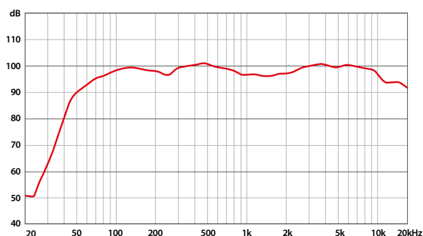
Frequenzgang:
