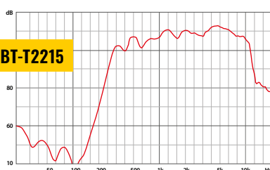
Frequenzgang:
