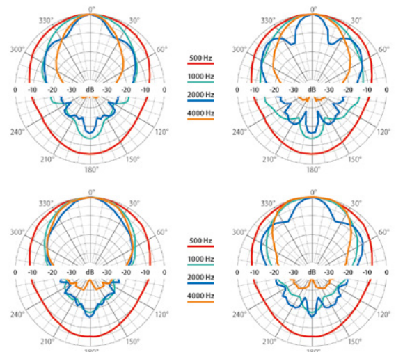
horizontal << Polardiagramm Richtcharakteristik >> vertikal
