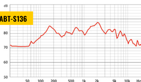
Frequenzgang:
