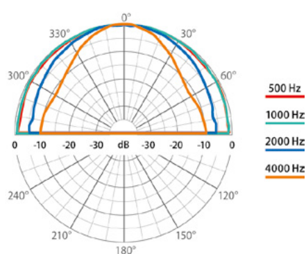
Polardiagramm Richtcharakteristik:
