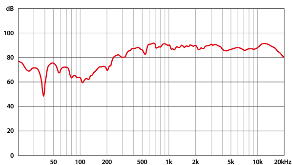
Frequenzgang:
