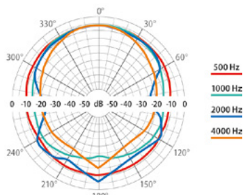
Polardiagramm Richtcharakteristik:
