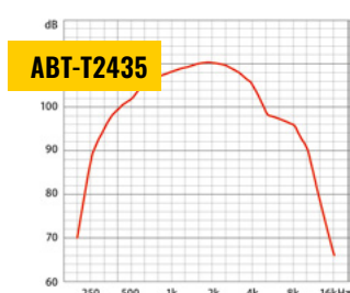
Frequenzgang:
