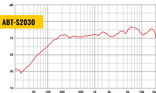
Frequenzgang:
