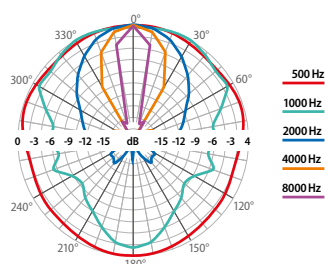
Polardiagramm Richtcharakteristik:
