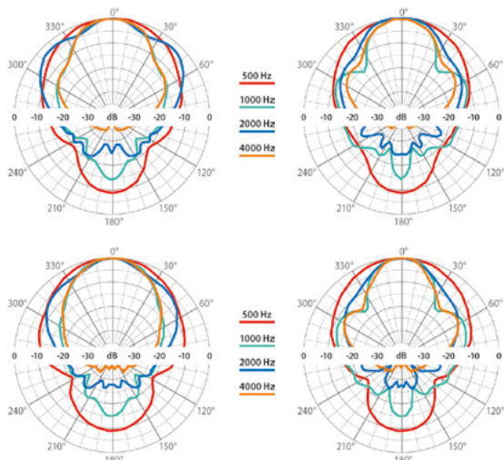
horizontal << Polardiagramm Richtcharakteristik >> vertikal
