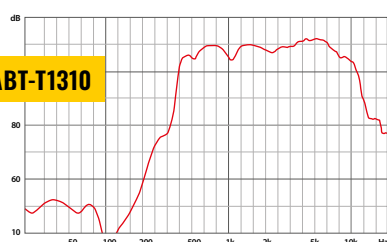
Frequenzgang:
