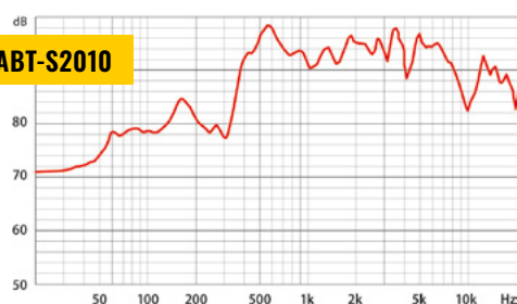
Frequenzgang:
