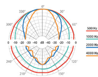
Polardiagramm Richtcharakteristik:
