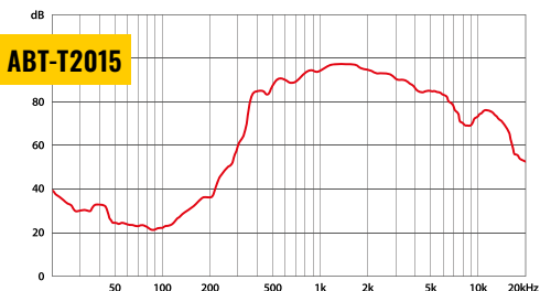
Frequenzgang:
