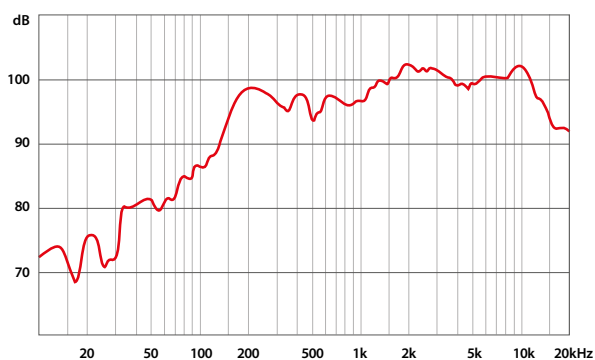
Frequenzgang:
