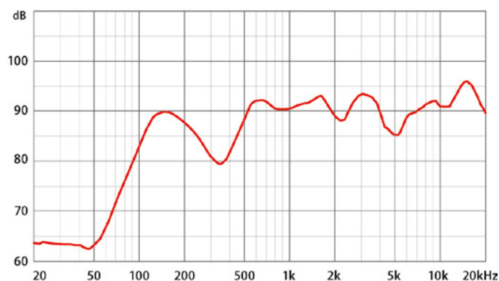
Frequenzgang:
