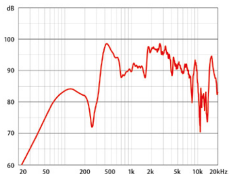
Frequenzgang:
