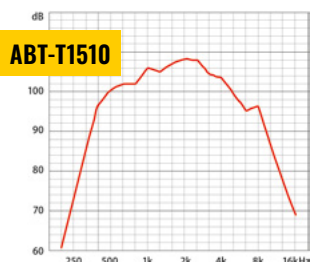
Frequenzgang:
